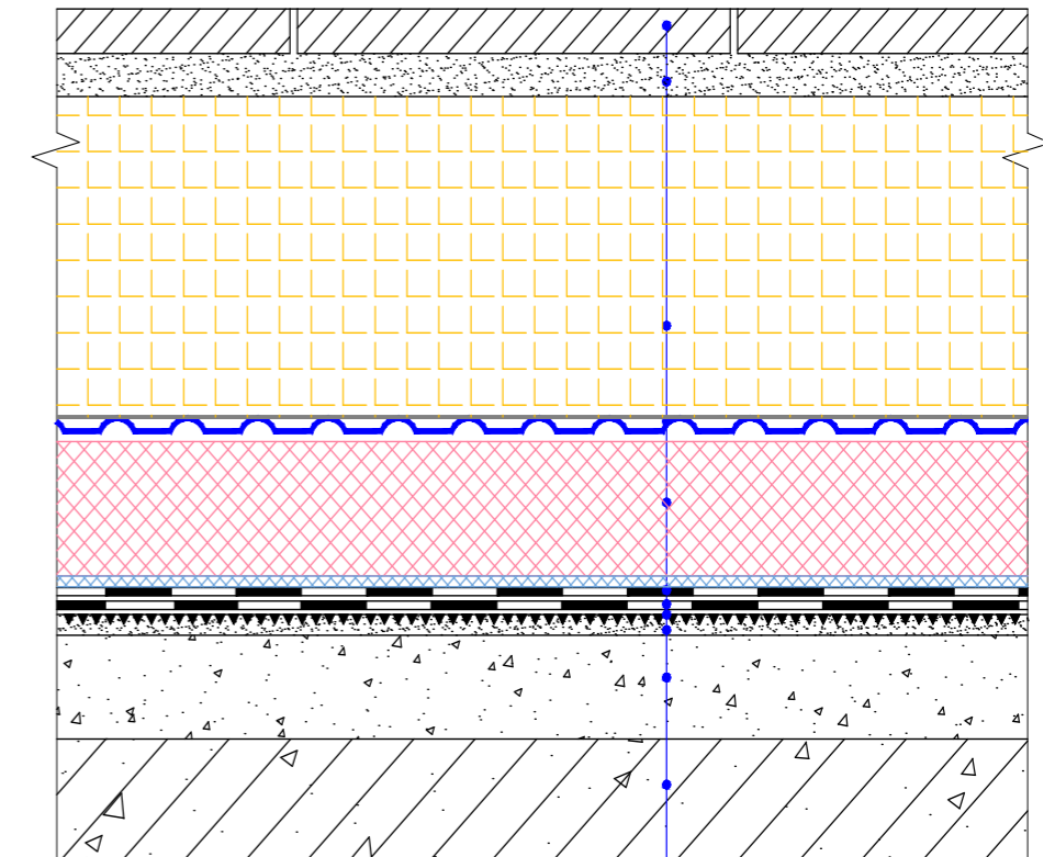
Рекомендация для устройства покрытия из бетонной плитки на стилобате
