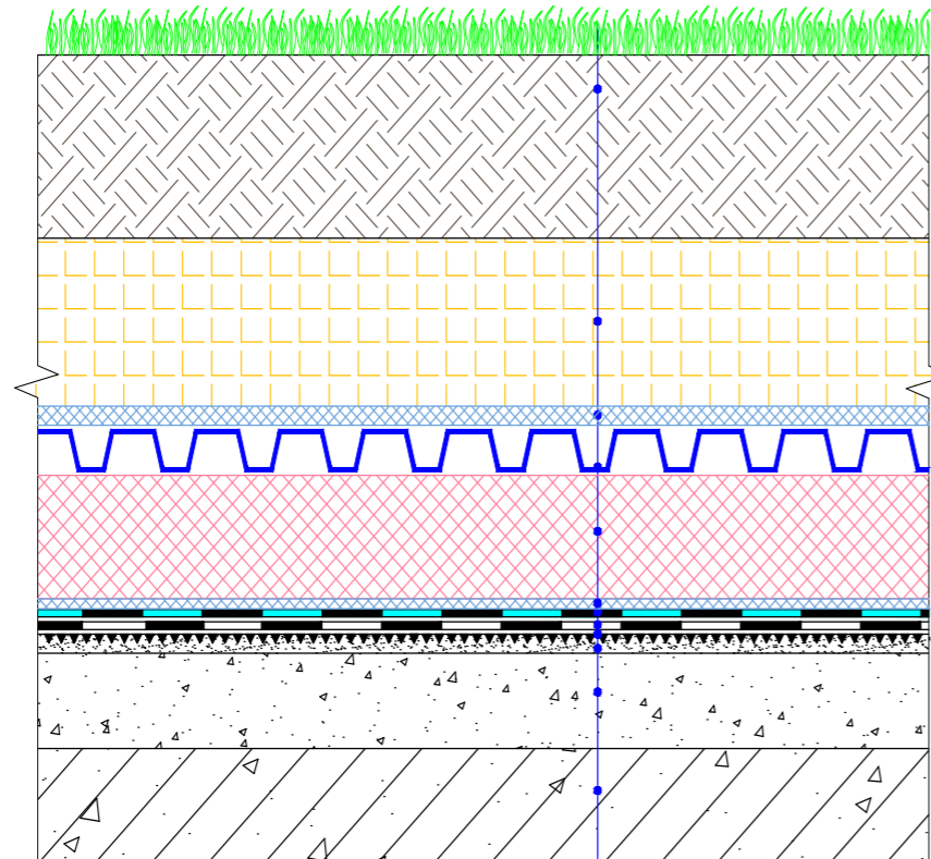
Рекомендация для устройства грунтового покрытия на стилобате
